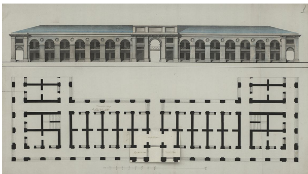
Рис. 4. Фасад гостиного двора, публикуется впервые (РГИА) Fig. 4. Facade of the Gostiny Dvor, published for the first time (RSHA)
