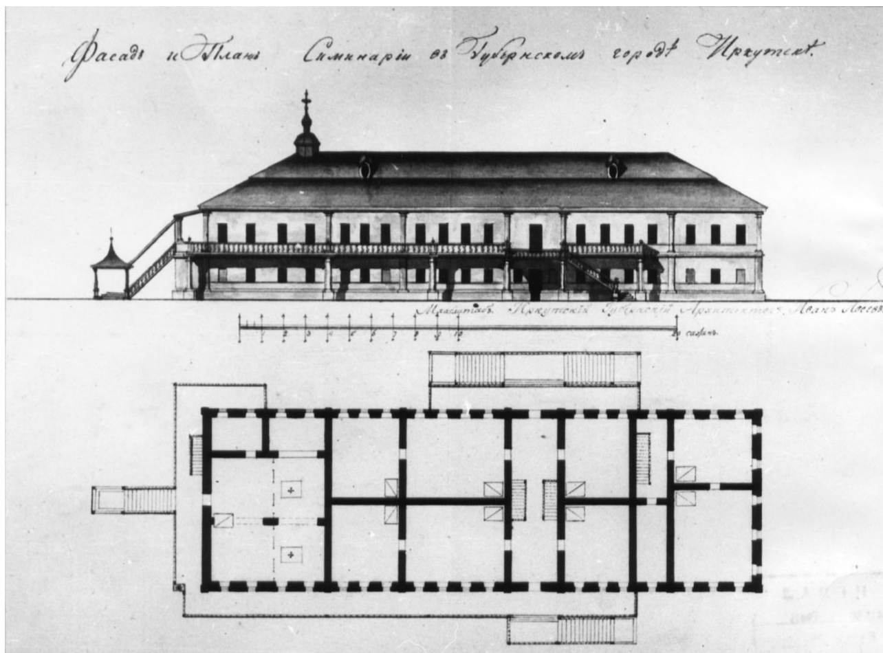
Рис. 1. Фасад и план семинарии в Иркутске (РГИА) Fig. 1. Facade and plan of the seminary in Irkutsk (Russian State History Archive, RSHA)
