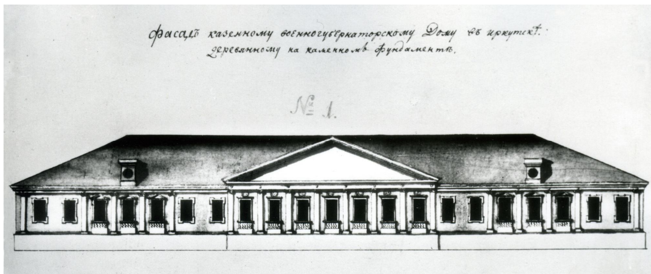
Рис. 2. Фасад казенного военно-губернаторского дома в Иркутске (рис. А. Лосева, РГИА) Fig. 2. The facade of the government-governor-military house in Irkutsk (fig. A. Losev, RSHA)
