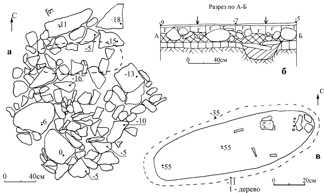
Рис. 9. Могильник Степушка-2. Объект 18а. План и профиль насыпи и погребения
