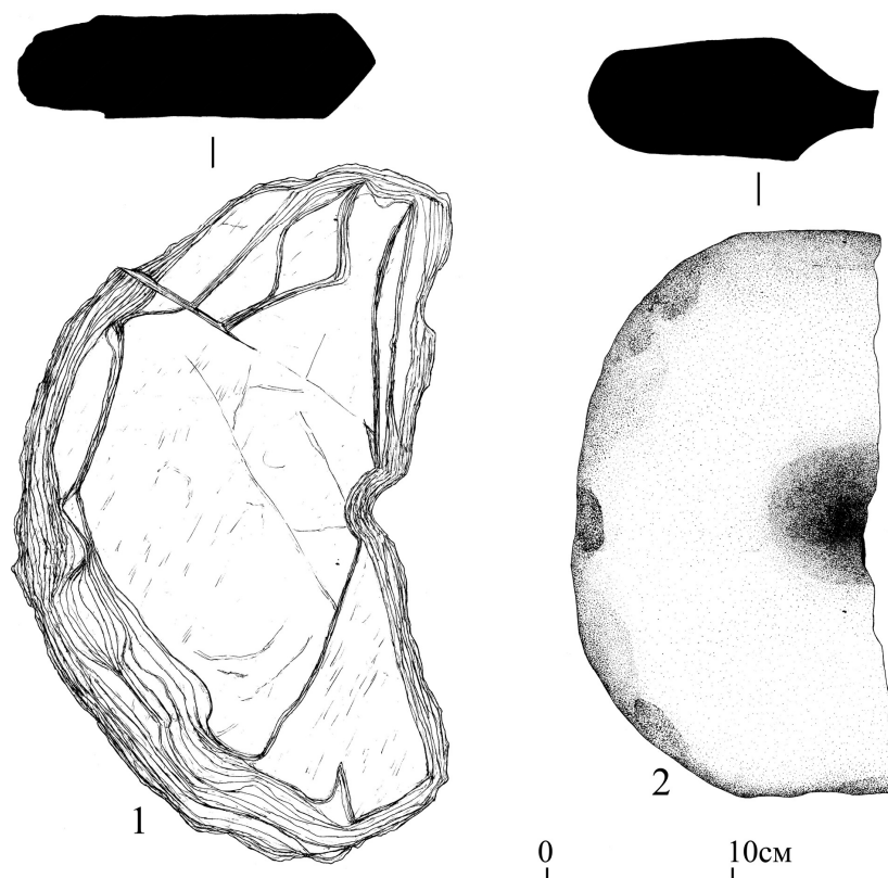
Рис. 14. Могильник Степушка-2. Заготовки жерновов ручных мельниц из насыпей объектов 21 (1), 22 (2).
