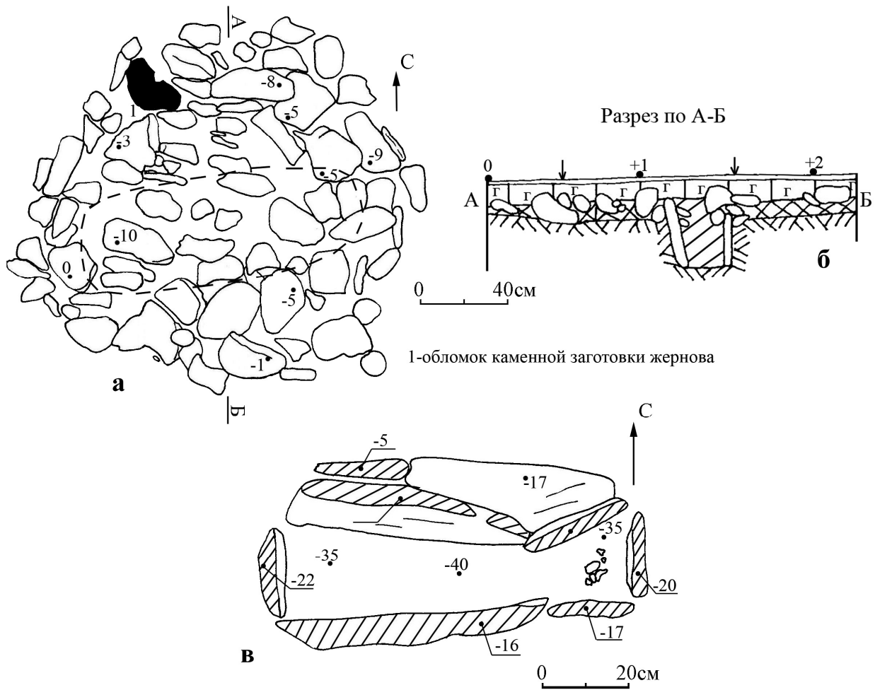
Рис. 11. Могильник Степушка-2. Объект 21. План и профиль насыпи и погребения
