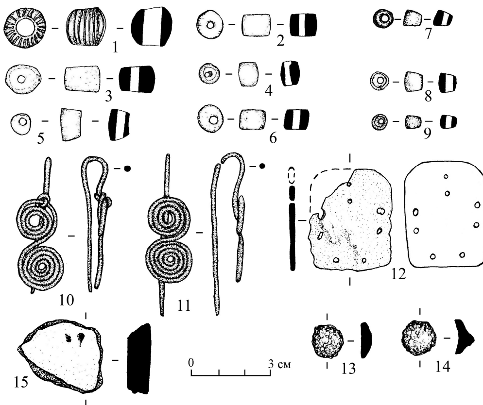
Рис. 13. Могильник Степушка-2. Инвентарь объектов 18а (7), 20 (1–6, 12–14), 21 (15), 22 (8–11): 1–9 – стеклянные и каменные бусины; 10–11 – бронзовые серьги со щитком в виде двух концентрических спиралей; 12 – железная панцирная пластина и ее реконструкция; 13, 14 – железные бляшки; 15 – фрагмент керамики
