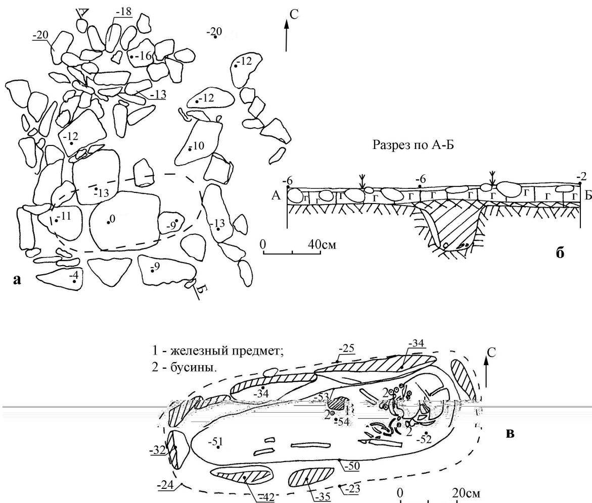
Рис. 10. Могильник Степушка-2. Объект 20. План и профиль насыпи и погребения
