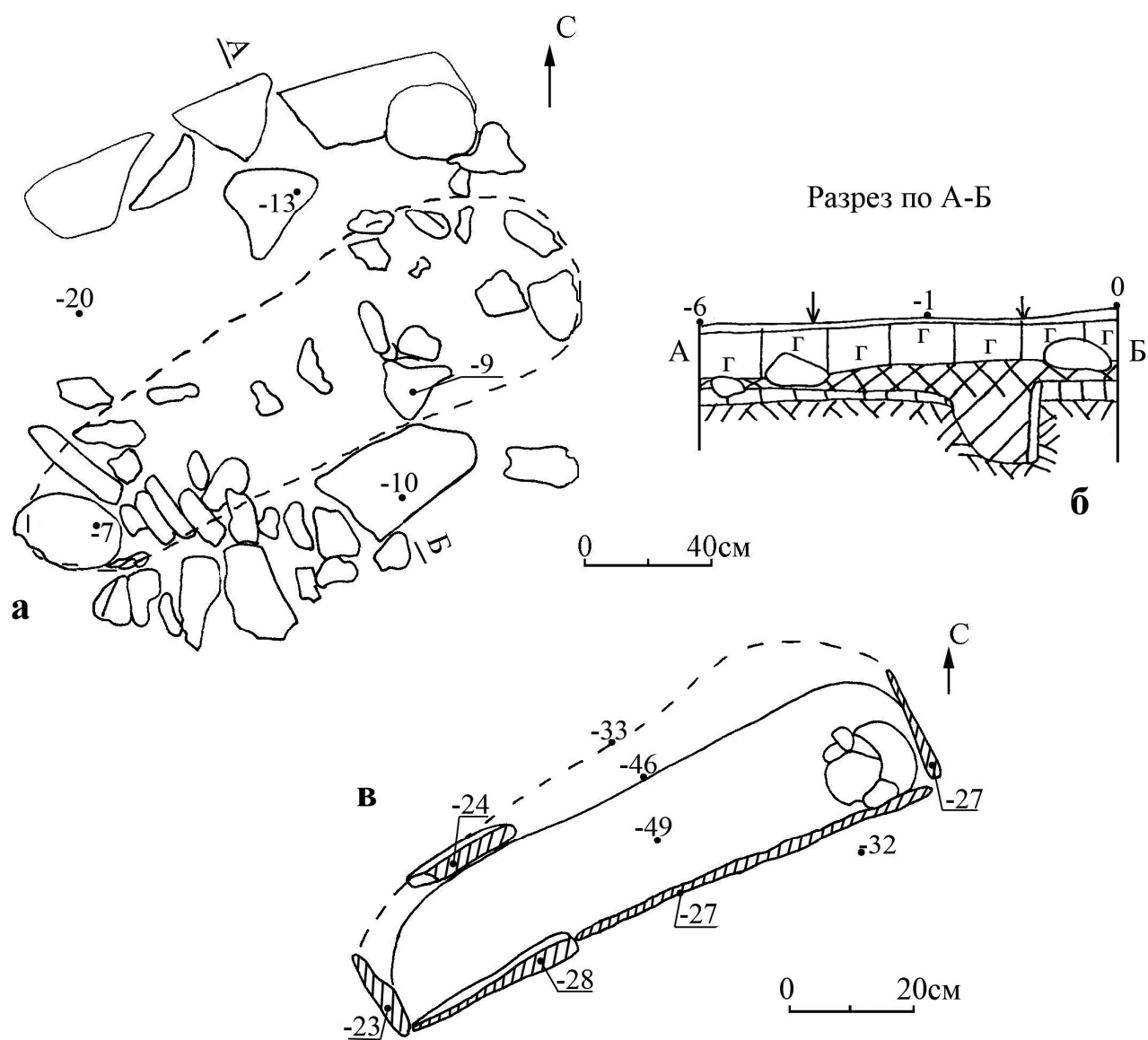
Рис. 6. Могильник Степушка-2. Объект 18. План и профиль насыпи и погребения
